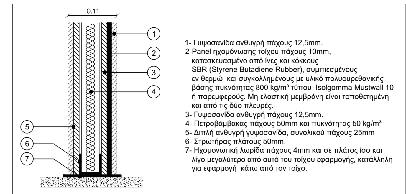
ΚΑΤΑΣΚΕΥΗ ΤΟΙΧΟΥ ΑΠΟ ΓΥΨΟΣΑΝΙΔΑ κλίμακα 1:5
