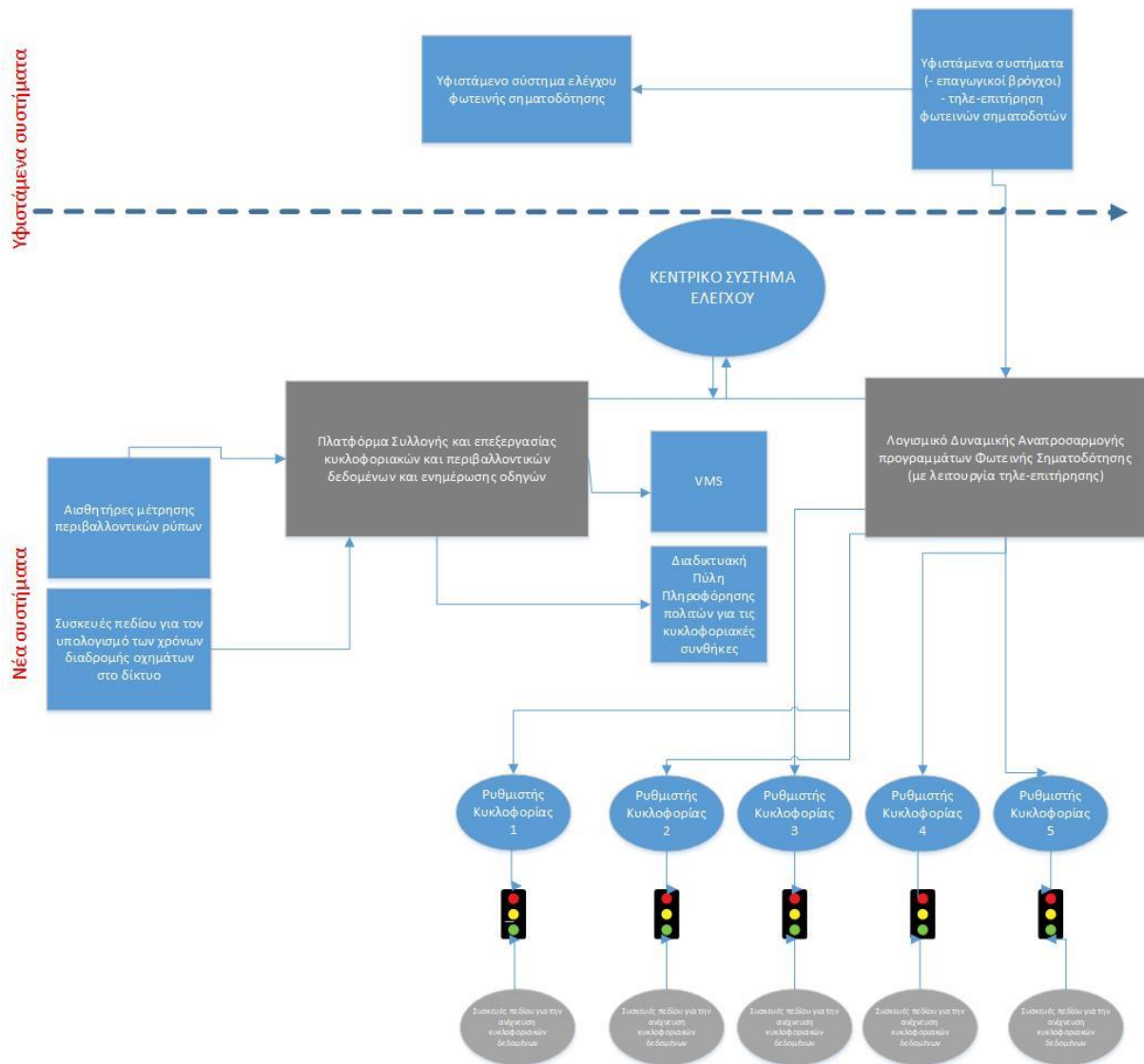
Διάγραμμα 1: ΑΡΧΙΤΕΚΤΟΝΙΚΗ ΣΥΣΤΗΜΑΤΟΣ
