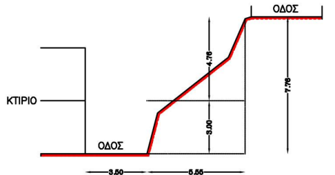
ΥΦΙΣΤΑΜΕΝΗ ΚΑΤΑΣΤΑΣΗ ΤΟΜΗ Α ΚΛ: 1/100
