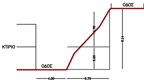
ΥΦΙΣΤΑΜΕΝΗ ΚΑΤΑΣΤΑΣΗ ΤΟΜΗ Β ΚΛ: 1/100
