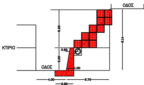
ΠΡΟΤΑΣΗ ΑΝΤΙΣΤΗΡΣΗΣ ΤΥΠΙΚΗ ΤΟΜΗ ΚΛ: 1/100
