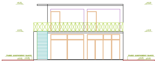
ΒΟΡΕΙΑ ΟΨΗ
