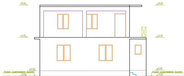
ΝΟΤΙΑ ΟΨΗ
