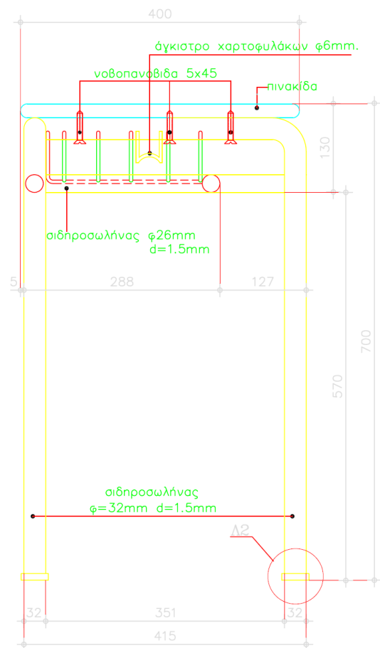
ΠΛΑΓΙΑ ΟΨΗ ΚΑΙΜΑΚΑ 1:5
