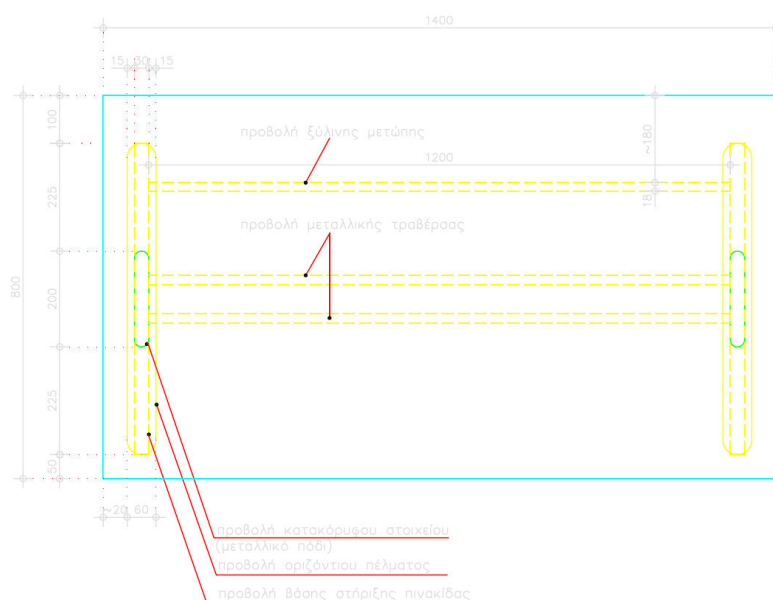
ΚΑΤΟΨΗ ΓΡΑΦΕΙΟΥ Η/Υ ΚΛ. 1:10
