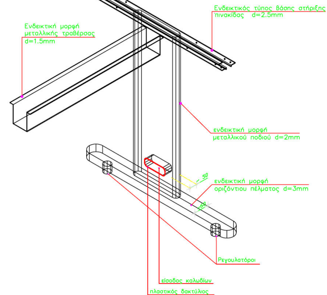
ΕΝΔΕΙΚΤΙΚΗ ΜΟΡΦΗ ΜΕΤΑΛΛΙΚΩΝ ΣΤΟΙΧΕΙΩΝ ΤΟΥ ΓΡΑΦΕΙΟΥ Η/Υ
