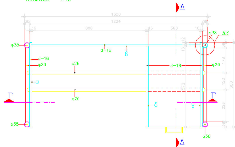
ΟΡΙΖΟΝΤΙΑ ΤΟΜΗ Β-Β ΚΑΙΜΑΚΑ 1:10
