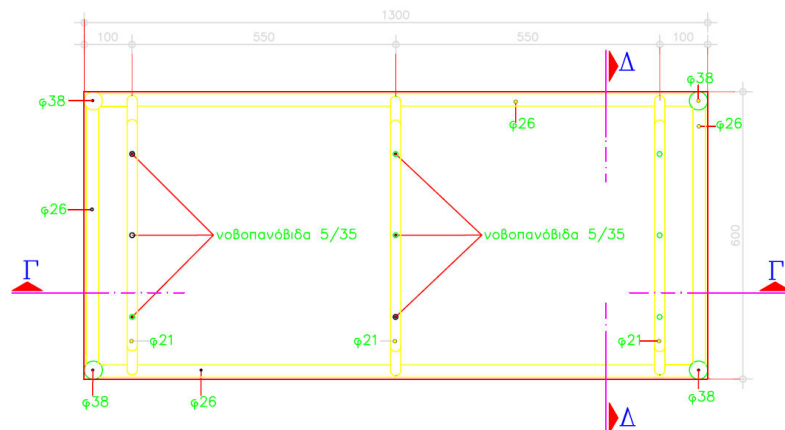
ΚΑΤΟΨΗ ΓΙΑ ΤΟΝ ΜΕΤΑΛΛΙΚΟ ΣΚΕΛΕΤΟ (Α-Α) ΚΑΙΜΑΚΑ 1:10
