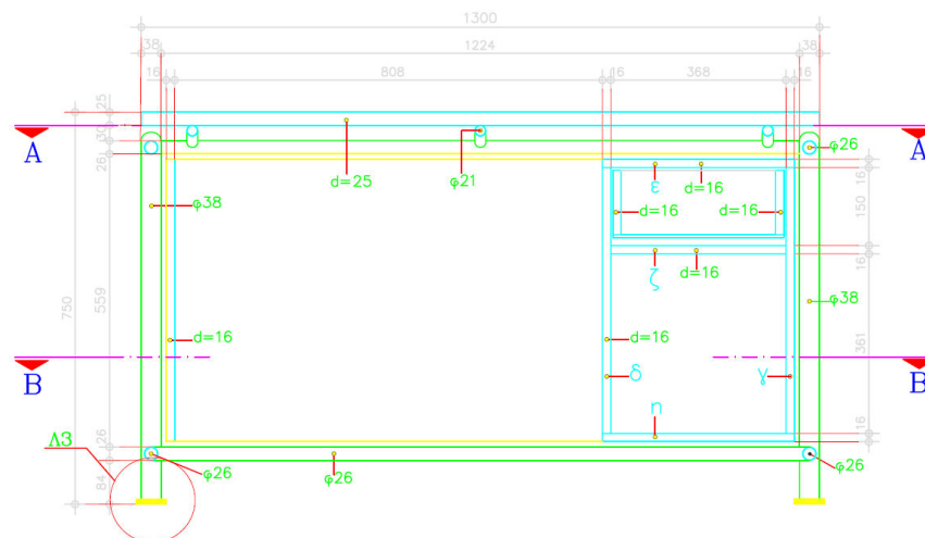
ΤΟΜΗ Γ-Γ ΚΑΙΜΑΚΑ 1:10
