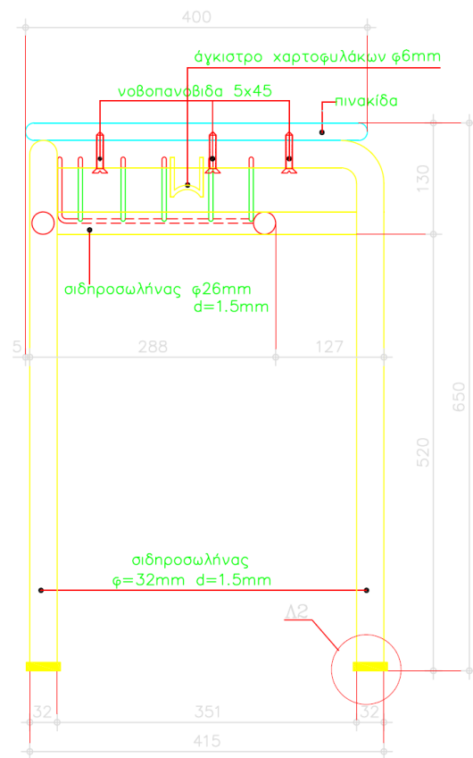
Π Λ Α Γ Γ Ι Α Ο Ψ Η ΚΛΙΜΑΚΑ 1:5
