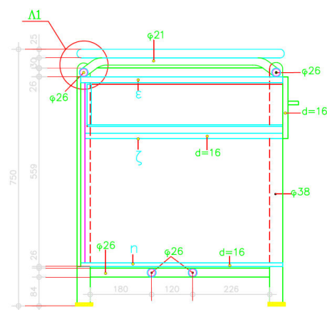
ΤΟΜΗ Δ-Δ ΚΑΙΜΑΚΑ 1:10
