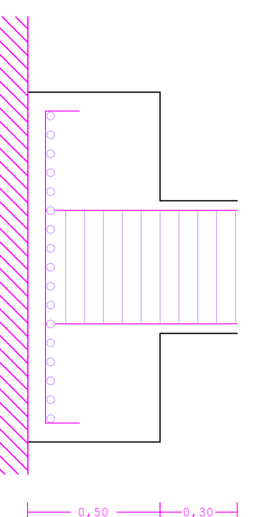
ΣΧΗΜΑΤΙΚΗ ΤΟΜΗ ΠΕΛΑΜΟΥ
