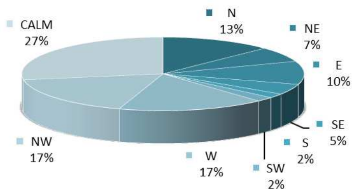
Εικόνα 1. Ετήσια Μέση Τιμή Συχνότητας κατεύθυνσης του ανέμου για τα έτη 1957-1997 (Ε.Μ.Υ – Χανια-Σούδα)
