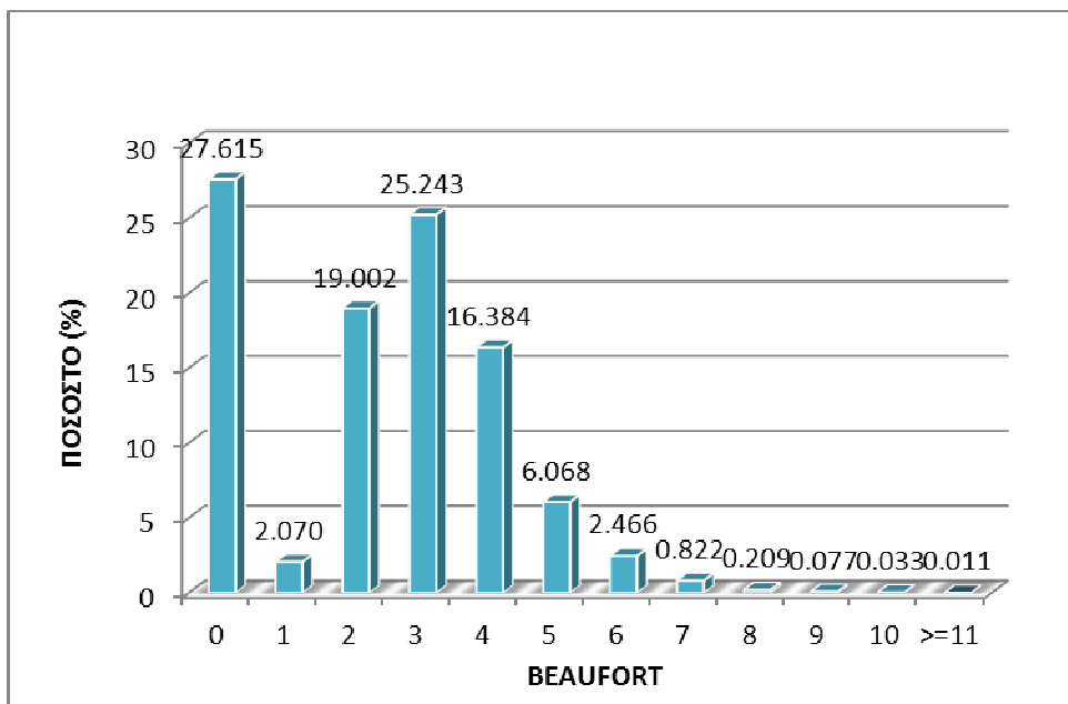
Εικόνα 2. Ετήσια Συχνότητα ανά τιμή beaufort του ανέμου για τα έτη 1957-1997 (Ε.Μ.Υ – Χανια-Σούδα)
