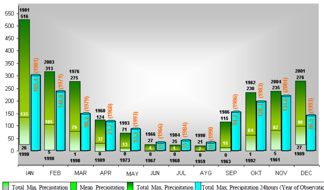
Εικόνα 4. Ραβδοδιάγραμμα ύψους υετού για τα έτη 1957-2004 (Ε.Μ.Υ – Χανια-Σούδα) [2]
