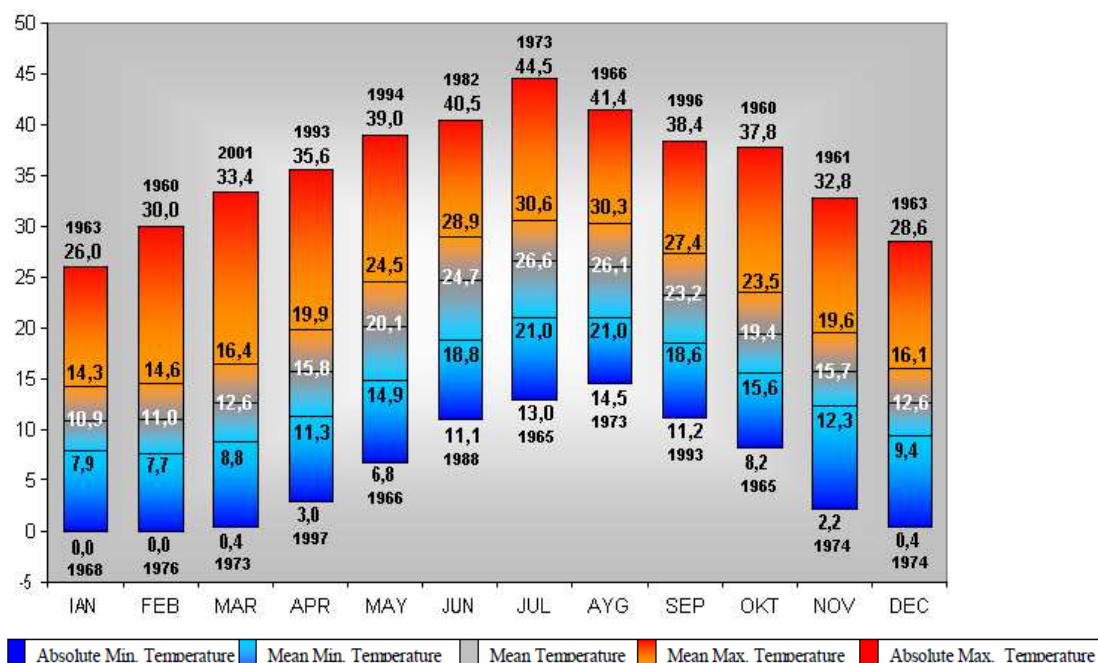
Εικόνα 3. Ραβδοδιάγραμμα θερμοκρασιών για τα έτη 1957-2004 (Ε.Μ.Υ – Χανια-Σούδα) [2]
