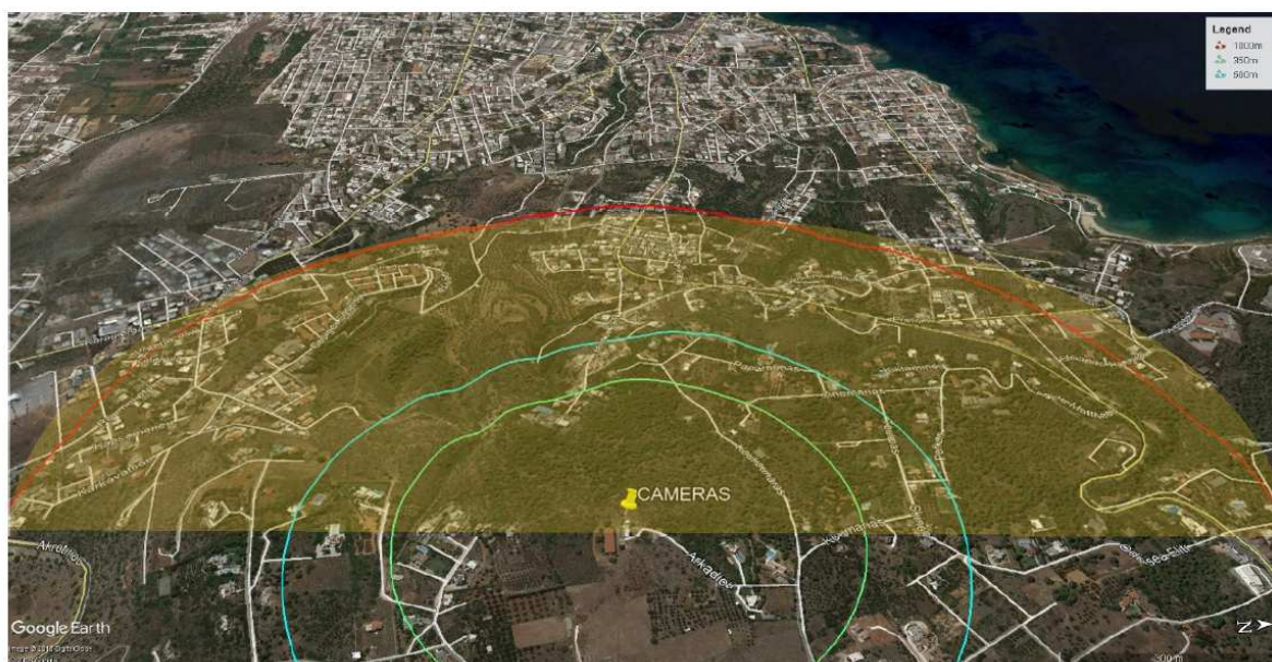
Εικόνα 11. Θέση εγκατάστασης της θερμικής κάμερας ανίχνευσης πυρκαγιάς και η περιοχή εφαρμογής της.
