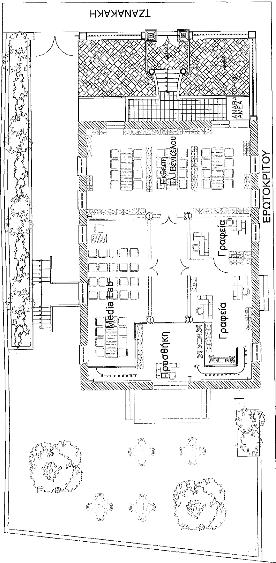
ΚΑΤΟΨΗ ΠΑΤΑΡΙΩΝ (ΠΡΟΣΘΗΚΗ) &Α' ΟΡΟΦΟΥ
