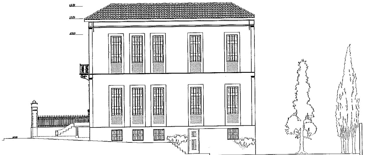
Δυτική Όψη
