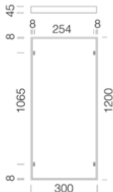
Εικόνα 3. Πλαίσιο στήριξης φωτιστικού σώματος.
