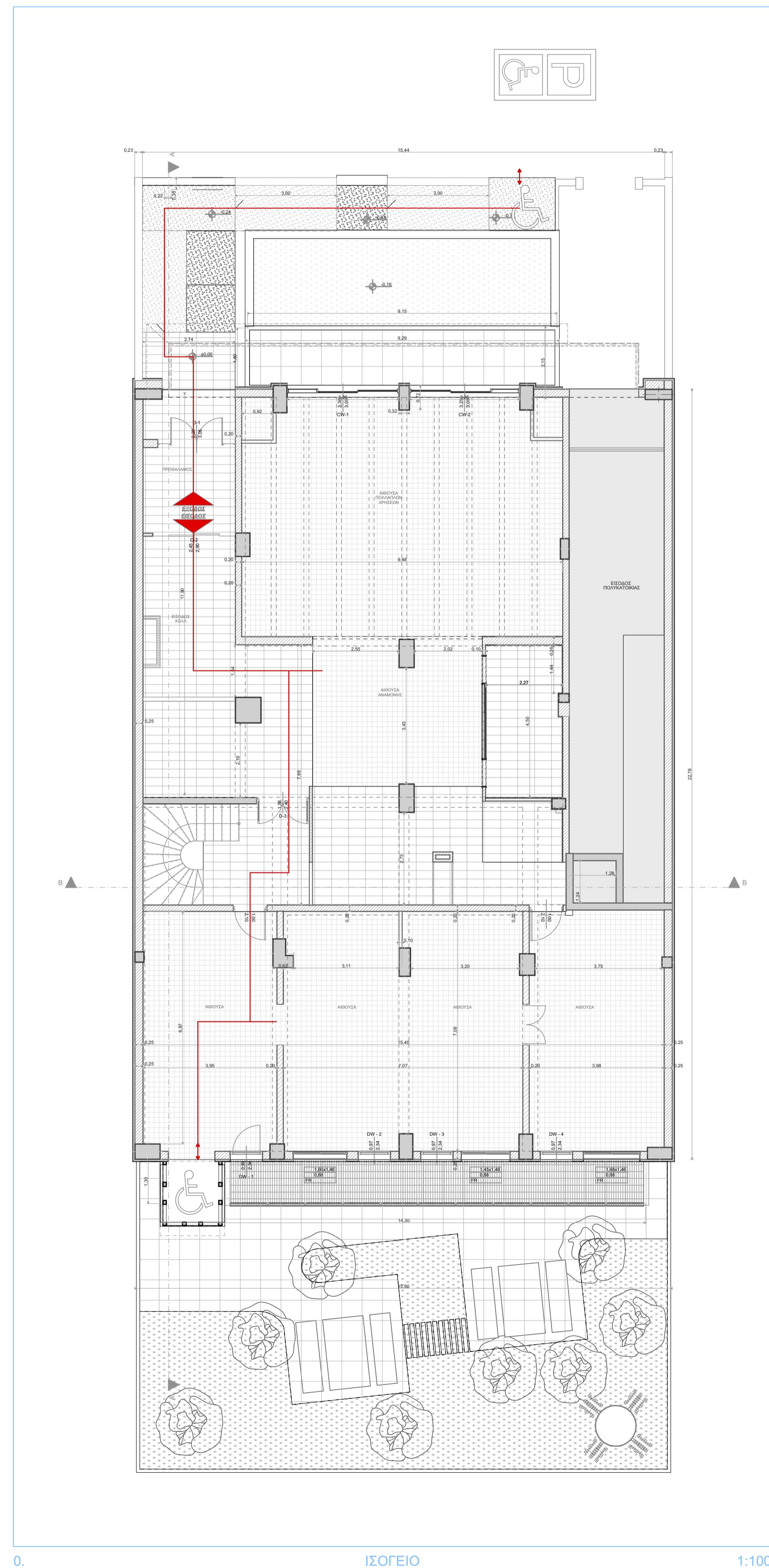
0. ΙΣΟΓΕΙΟ 1:100
