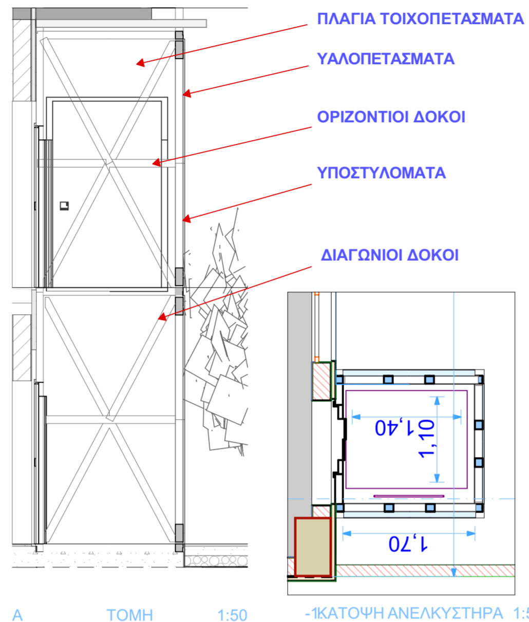
A ΤΟΜΗ 1:50
