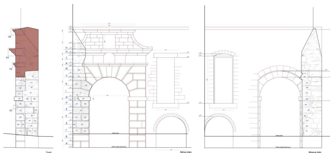
Εικόνα 2. Όψη και τομή πύλης
